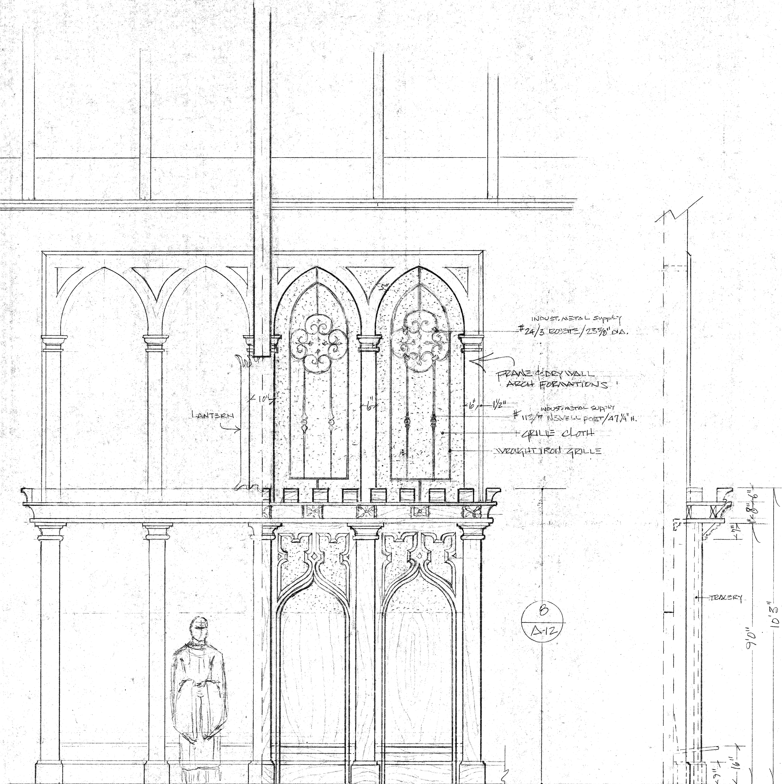
1 ELEVATION
