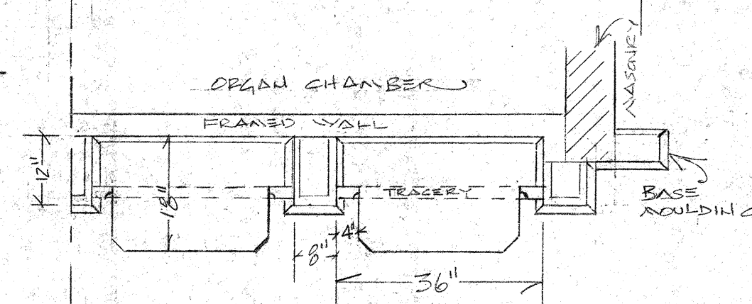
1 ELEVATION
